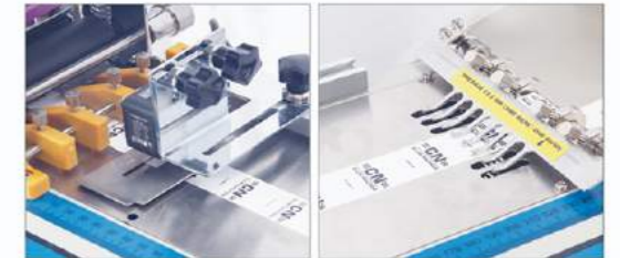
WJ100-B / 全自动电脑切带机 Automatic Belt Loop Cutter Series
